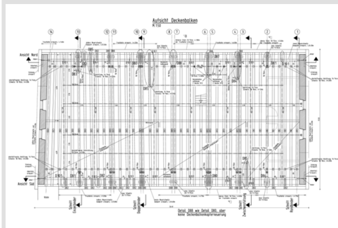
Sanierungszeichnungen / Ausführungszeichnungen Ing.-Büro Prof. Dr. R. Hempel & Partner, Köln
