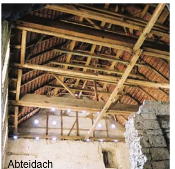
Abteidach
